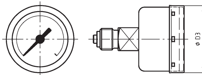
Typ 131.11 bakåtriktad utförande med kapsel
